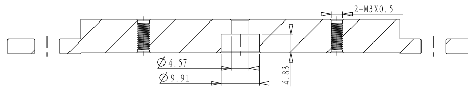
截面 A-A
