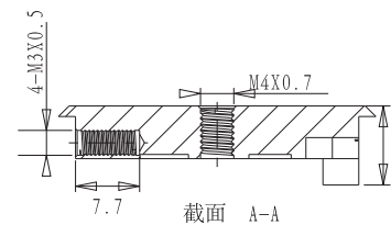
截面 A-A
