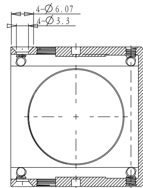
截面 A-A
