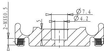
截面 A-A
