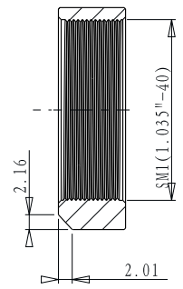
截面 A-A
