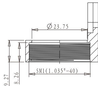
截面 A-A
