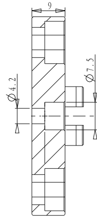
截面 A-A
