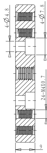
截面 B-B
