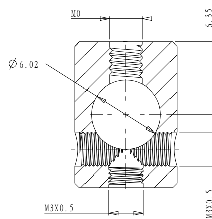
截面 A-A
