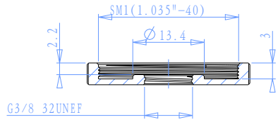
截面 A-A
