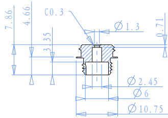
截面 C-C 比例 1.000
