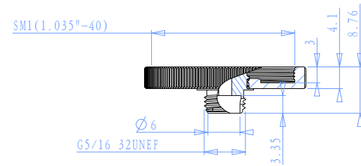
截面 A-A
