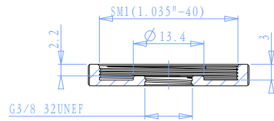
截面 A-A
