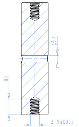
截面 A-A
