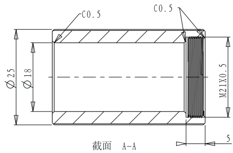
截面 A-A
