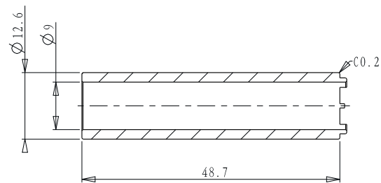
截面 A-A
