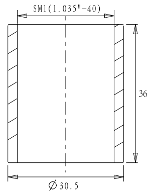
截面 A-A
