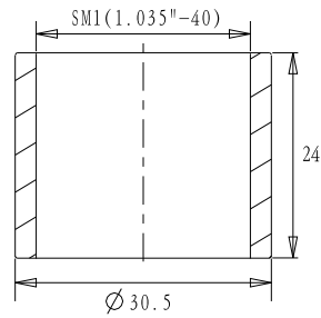
截面 A-A
