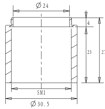
截面 A-A
