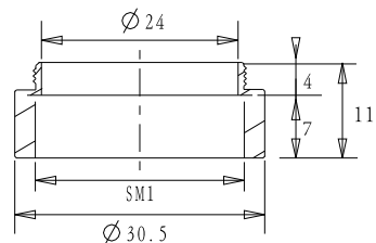
截面 A-A
