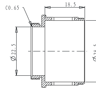
截面 A-A
